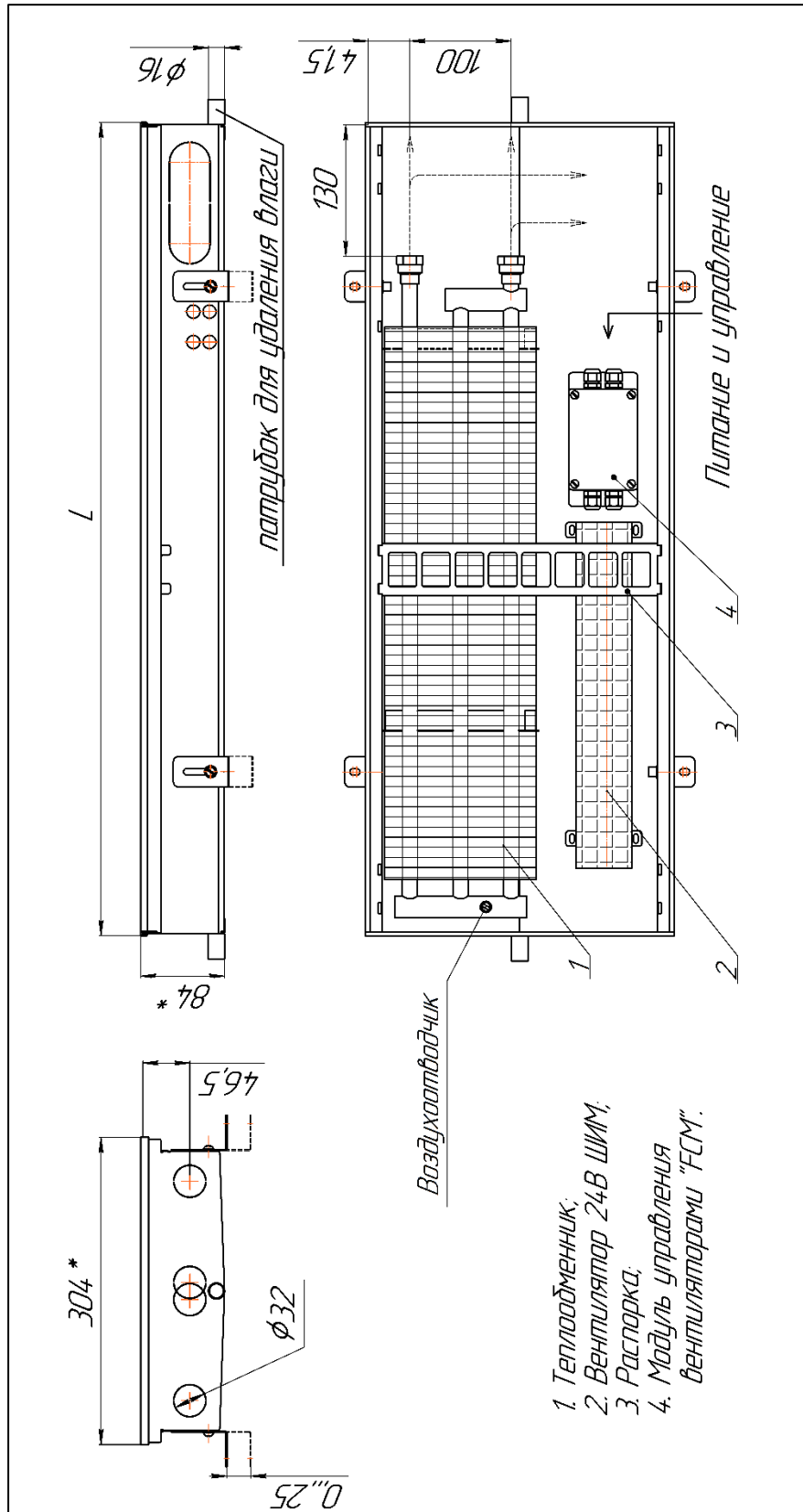
Монтажная схема
